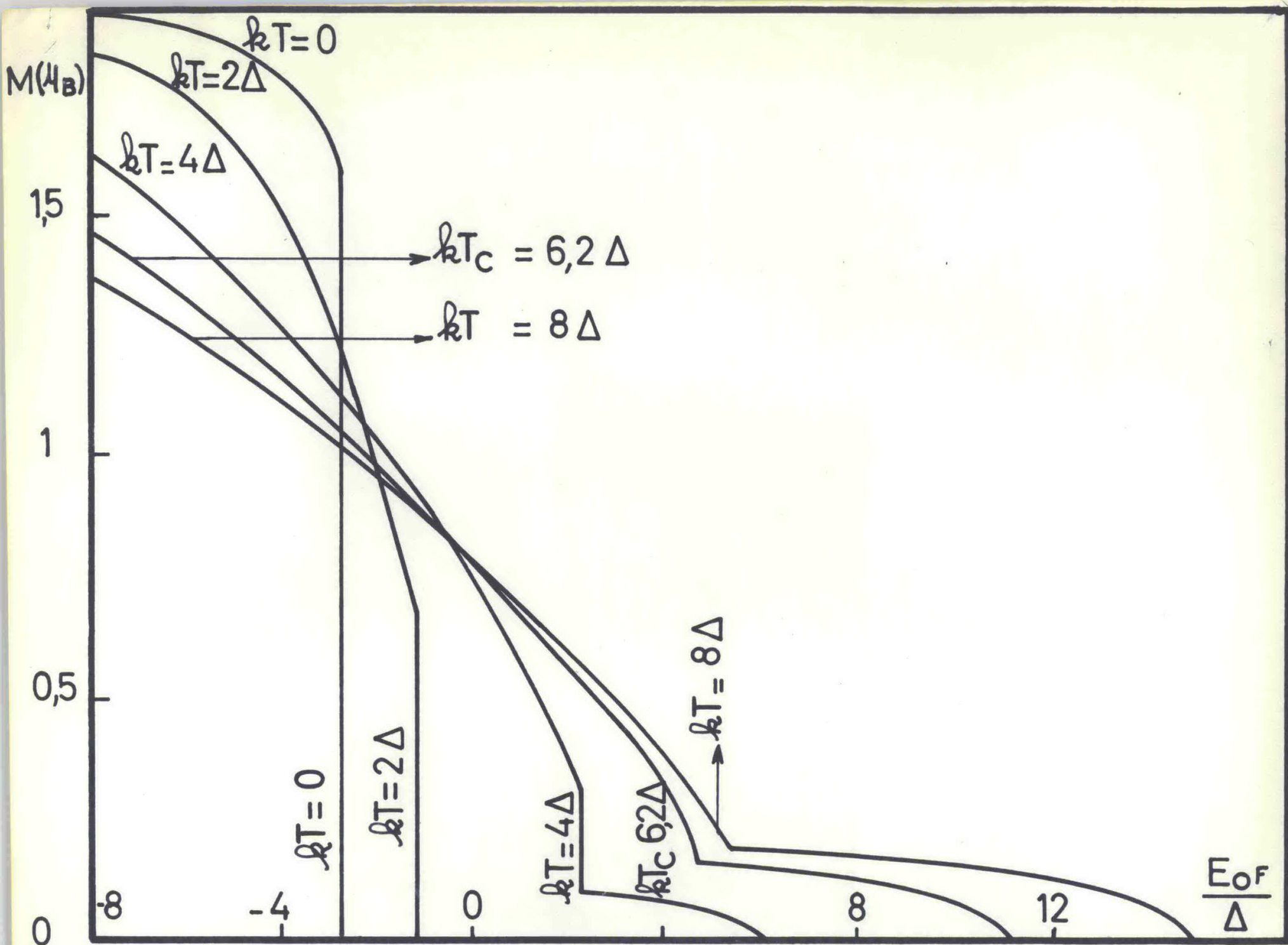
Fig-22: Moment magnétique \frac{U}{\Delta} = 250 - \frac{J}{\Delta} = 150
